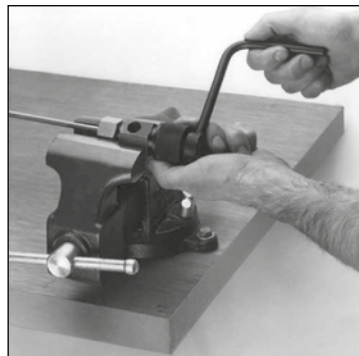
2. Снятие фаски
