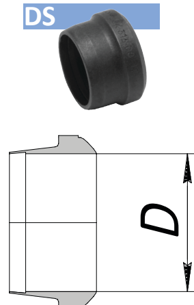
Врезное кольцо
