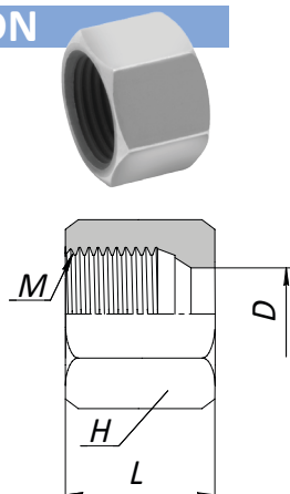
Гайка
